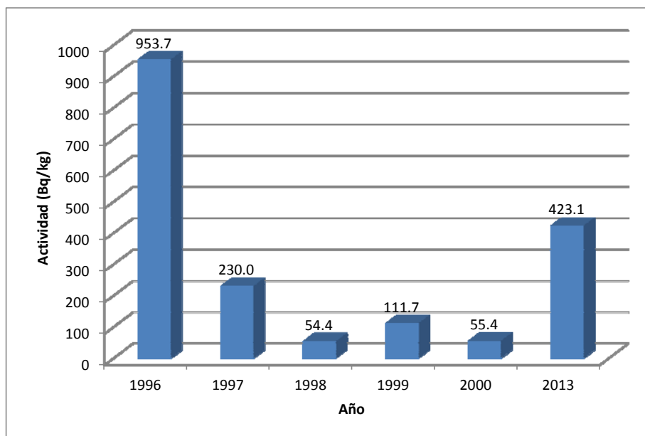
Figura 2. Actividad derivada de ^7\text{Be} en Usnea antarctica Du Rietz (1996-2013).
